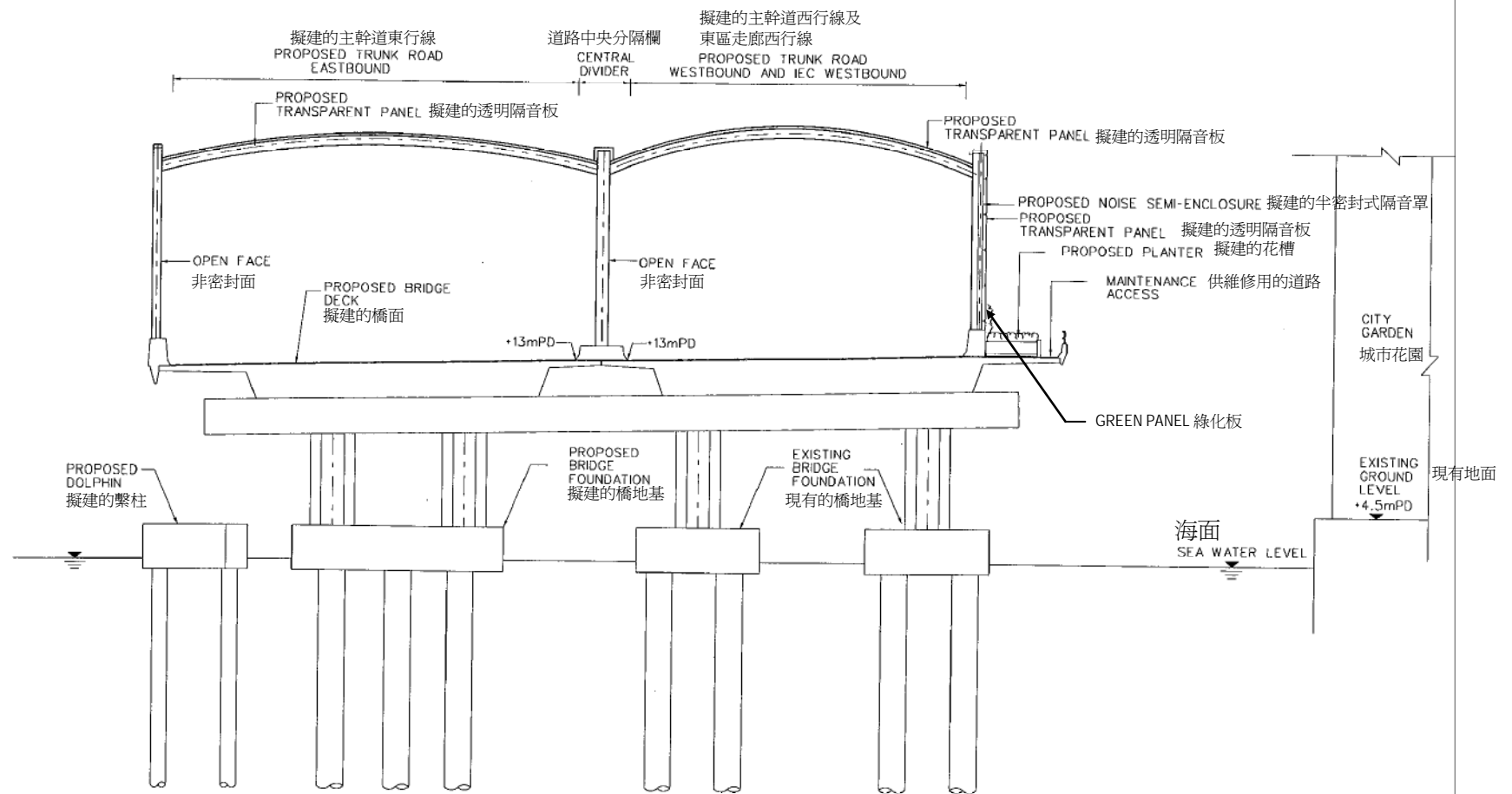
切面 C-C SECTION C-C
